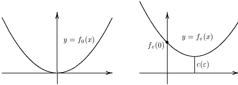
FIGURE 28.16. Lemma 28.5
