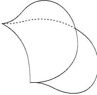
FIGURE 13.10. Cuspidal edge
